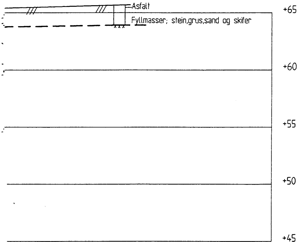
Profil B-B
