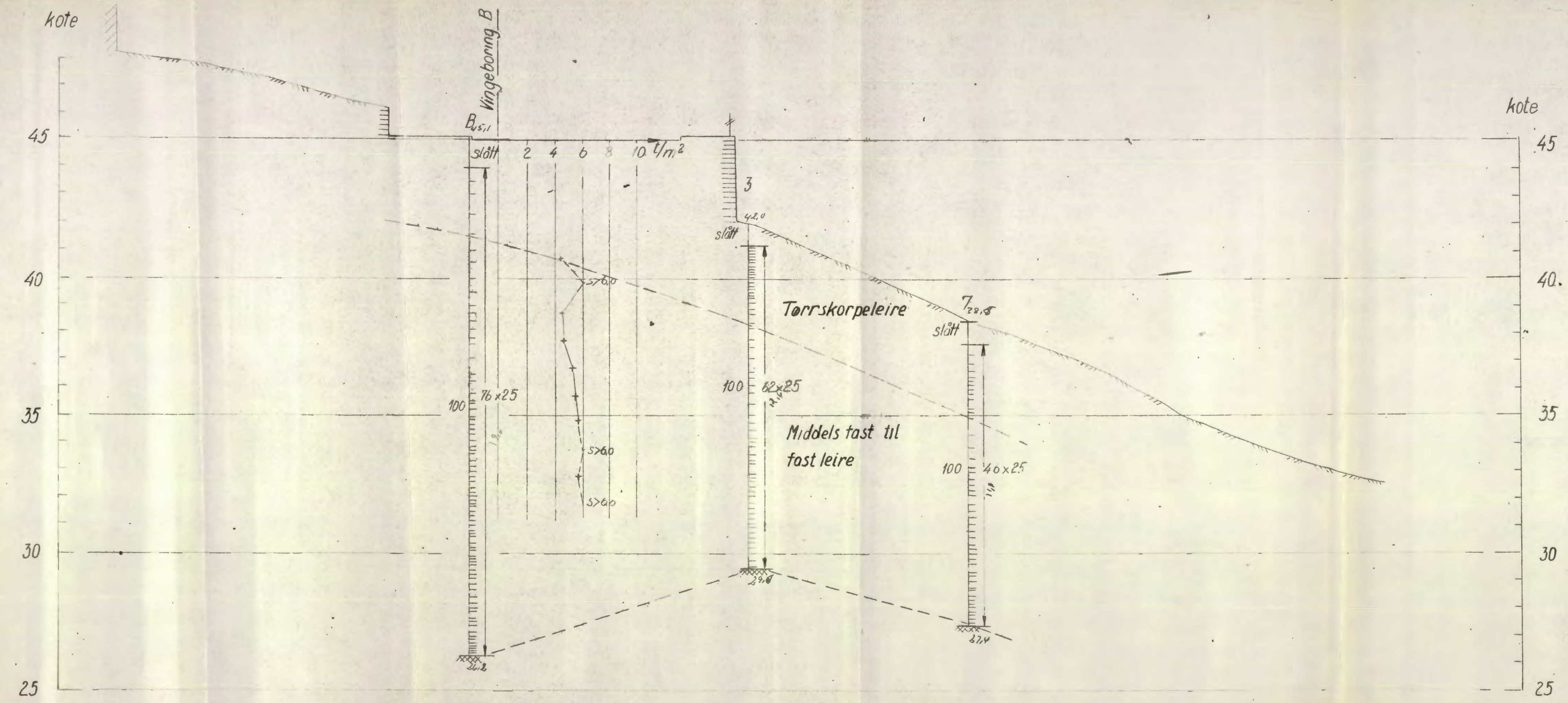
PROFIL IV Dreieboringer og vingeboringer ML=1:100 MH=1:100 Ant fjell Norges geotekniske institutt aug 54
