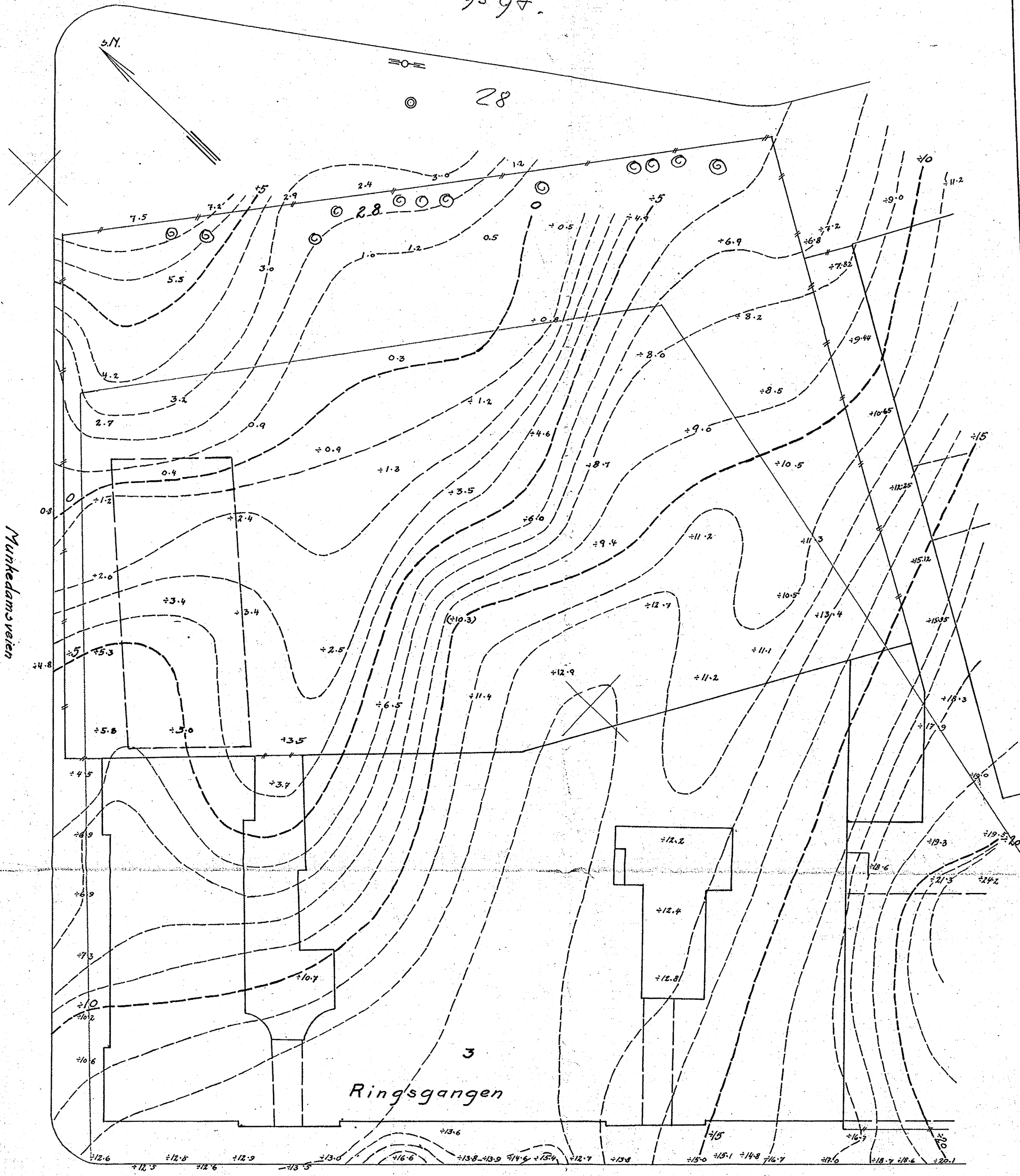
Grundboringskart over Bedstefarstomten M. 1:200 m.m.
