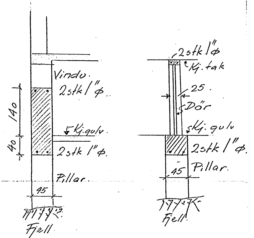
Snitt A-A 1:50
