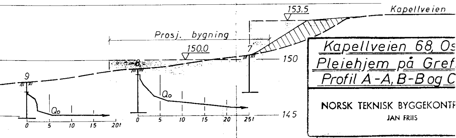
Profil C - C
