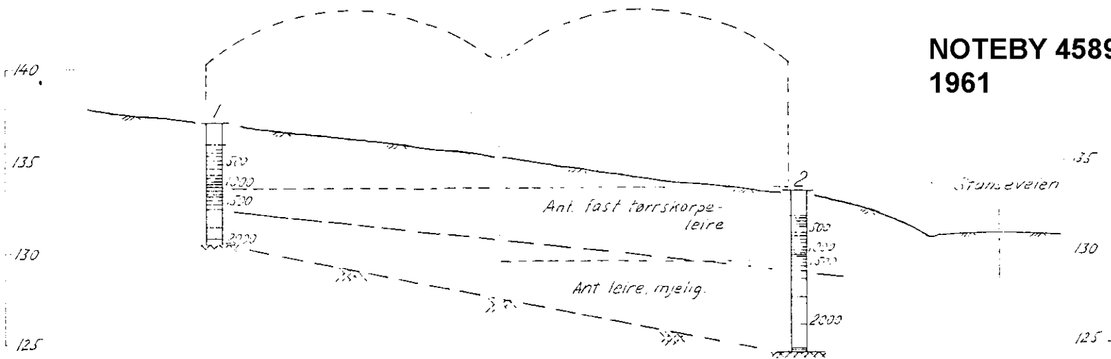
Profil A-A
