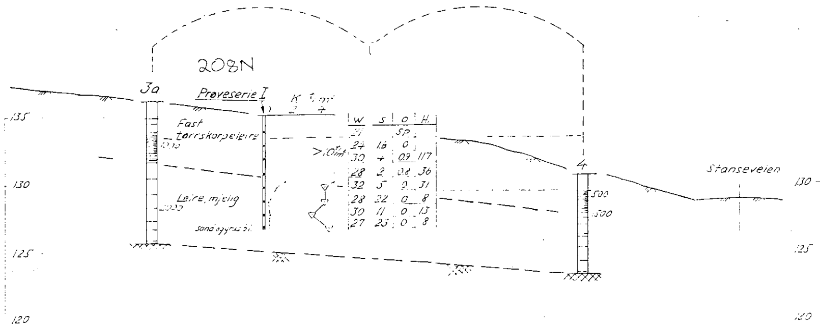
Profil B-B
