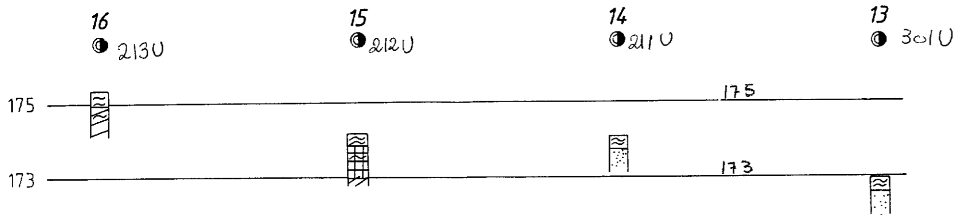
Profil A - A
