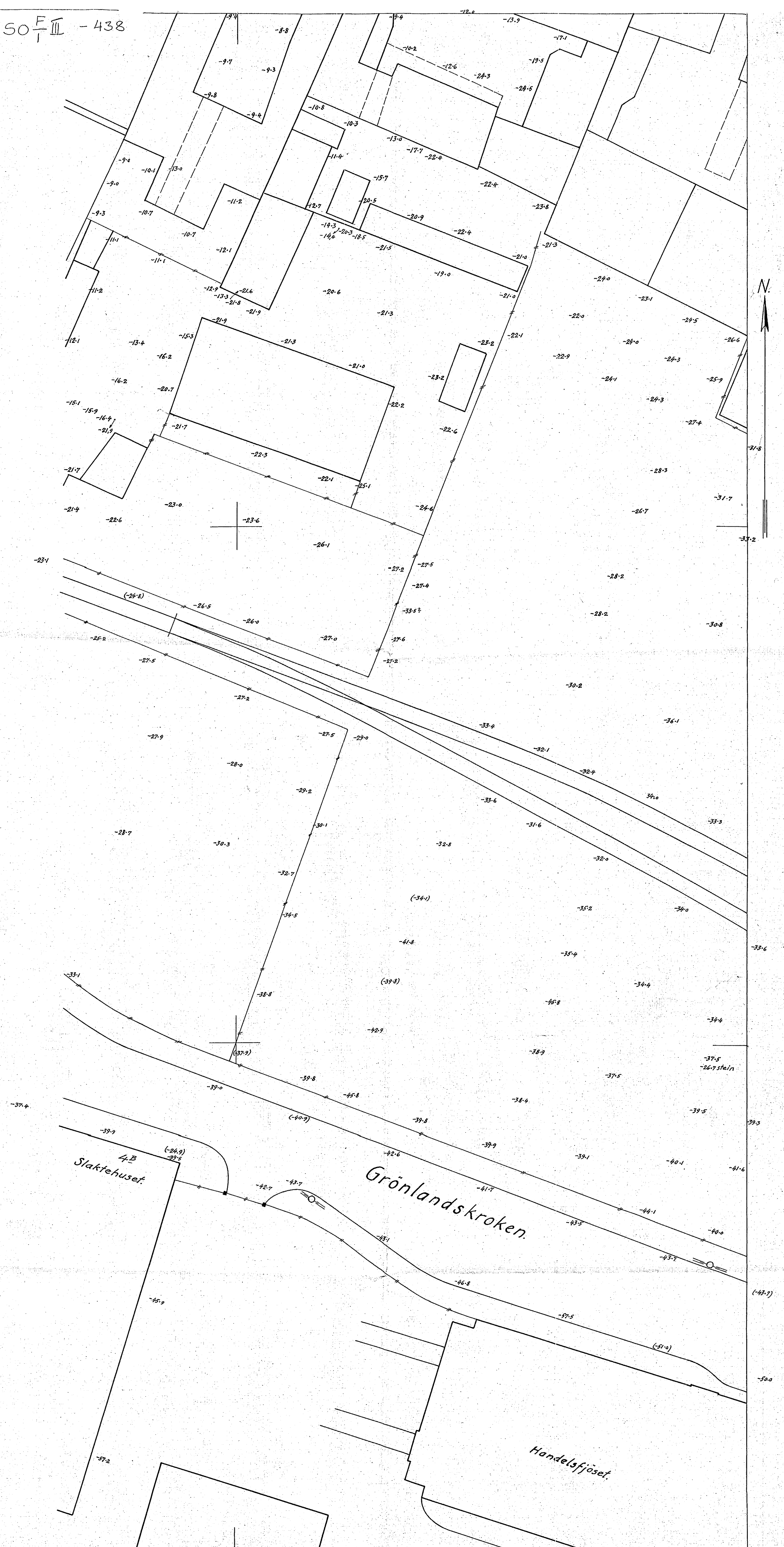
S.O. F III Bl. nr. 438. Grundboringskart M:1:200. Fert a jour 30-4-1927.
