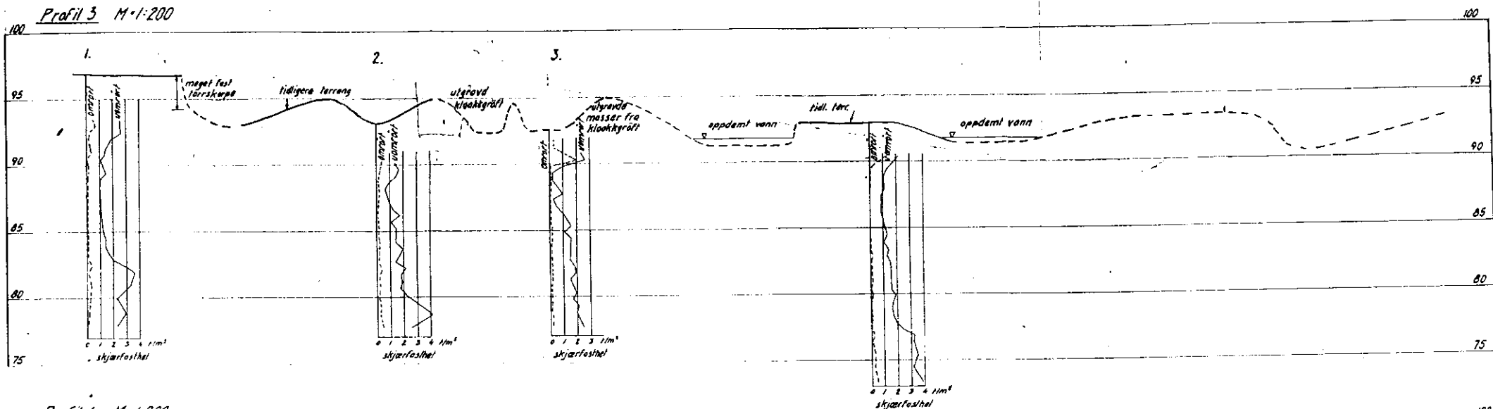
Profil 4 M=1:200
