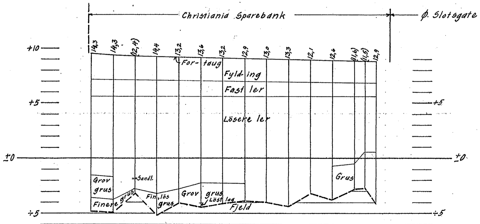
Profil gjennom boringer paa fortaug langs sydvestre væg
