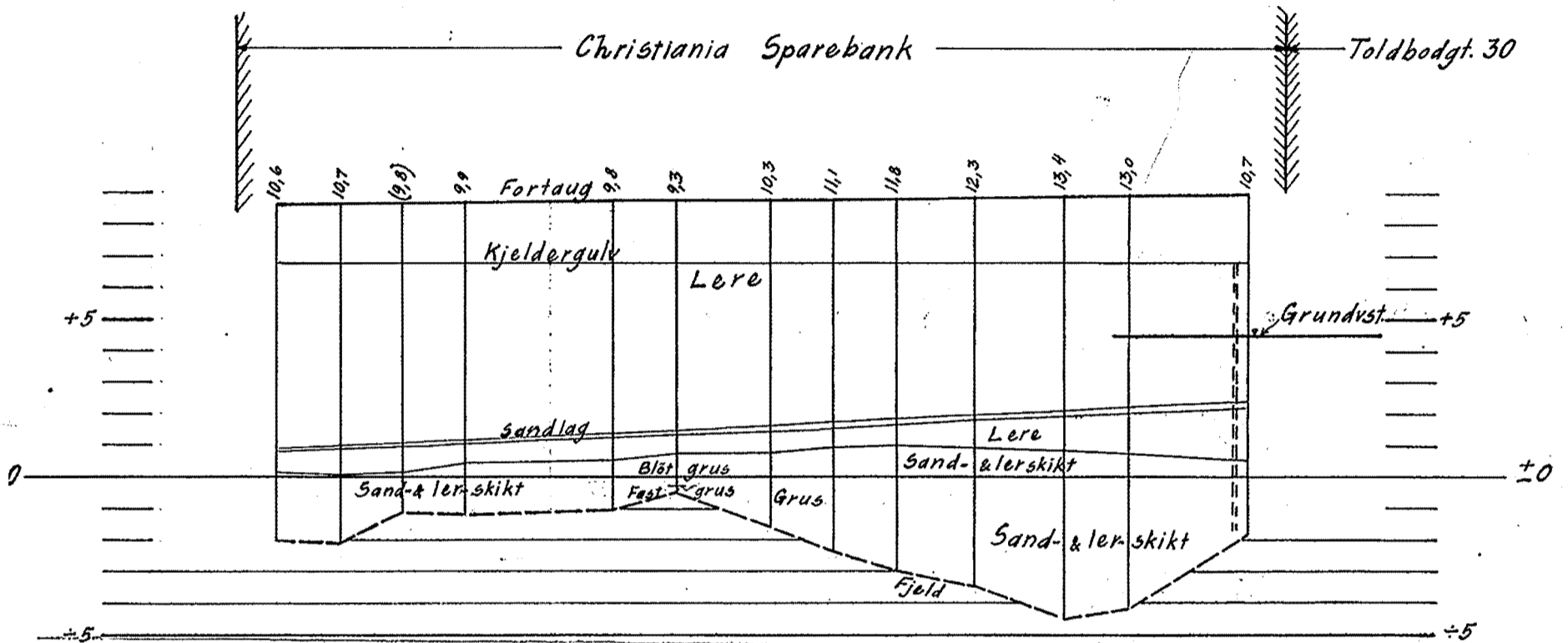
Profil gjennom boringer paa fortaug langs sydvestre væg
