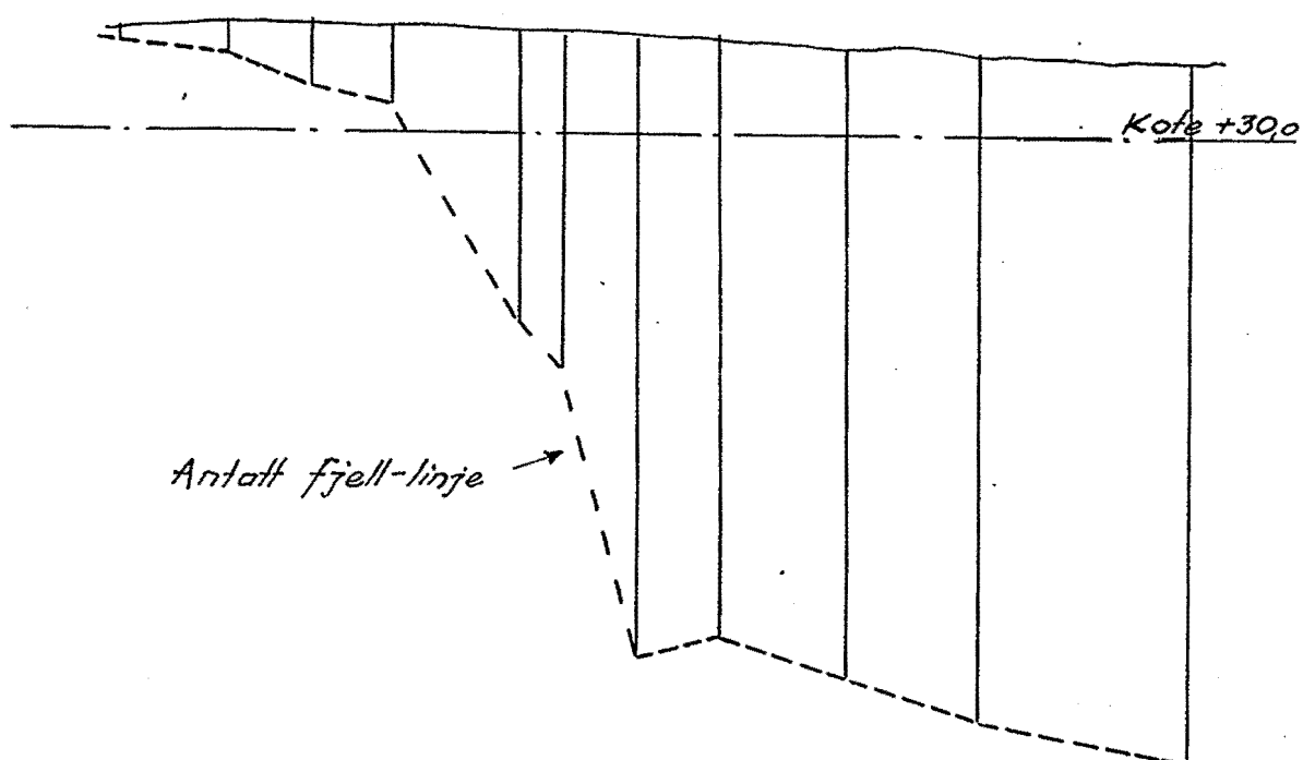
Profil 2-2.
