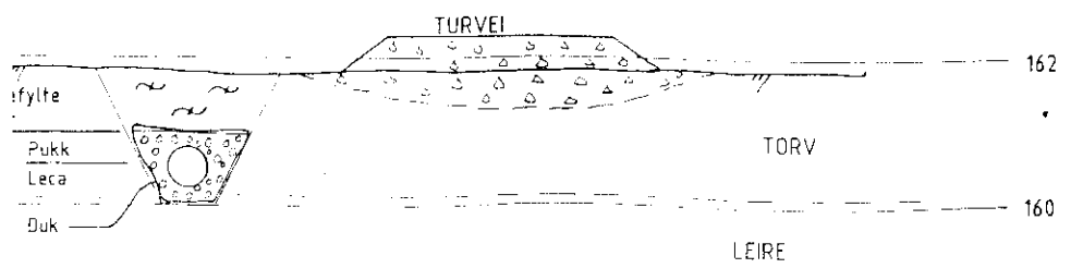
TVERRPROFIL M 1 : 100 PROFIL 7 + 55m
