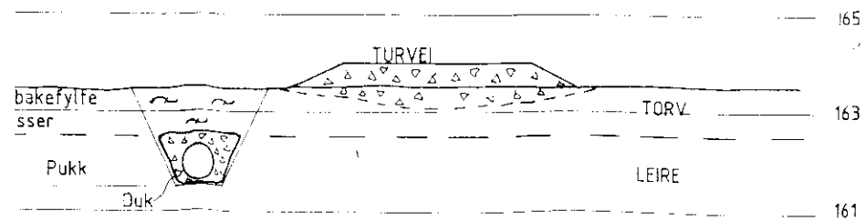
TVERRPROFIL M 1 : 100 PROFIL 6 + 30m
