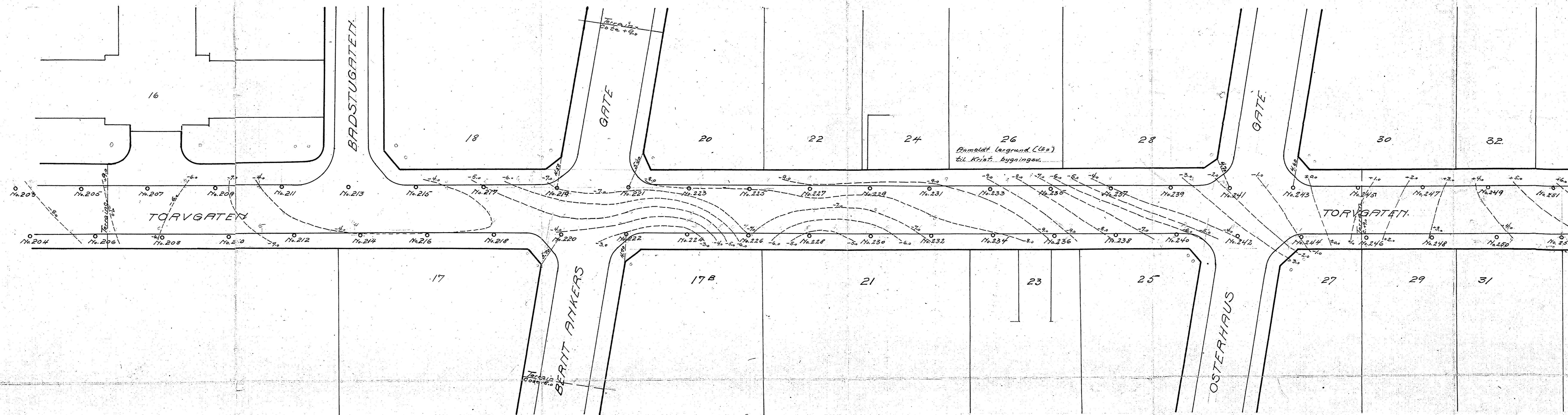
PROFIL EFTER BORHULLER 170204, 206--250, 252.
