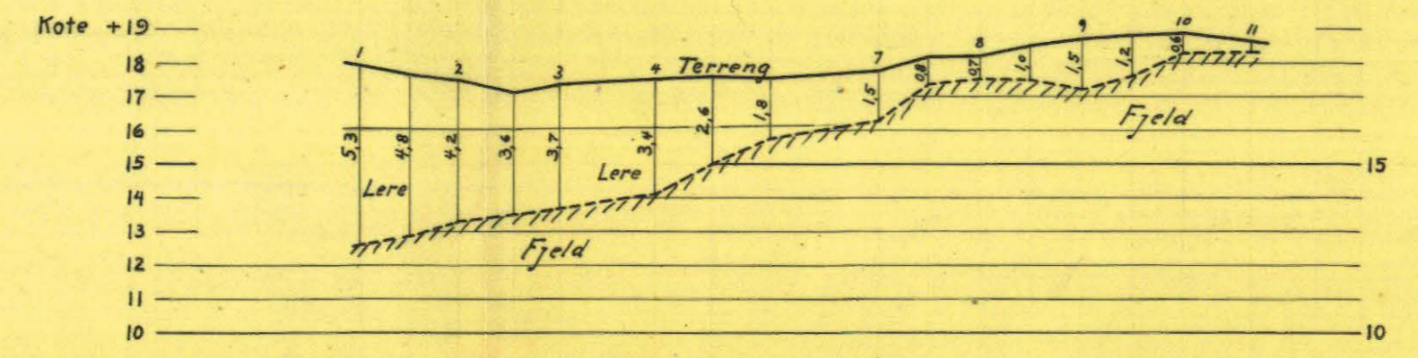
Profil langs boringerne H. og L. M. = 1:200.
