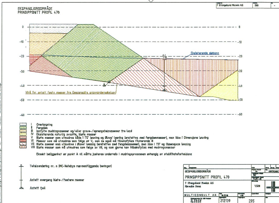
Figur 1 Prinsippssnitt profil 470 i ekspansjonsområdet
