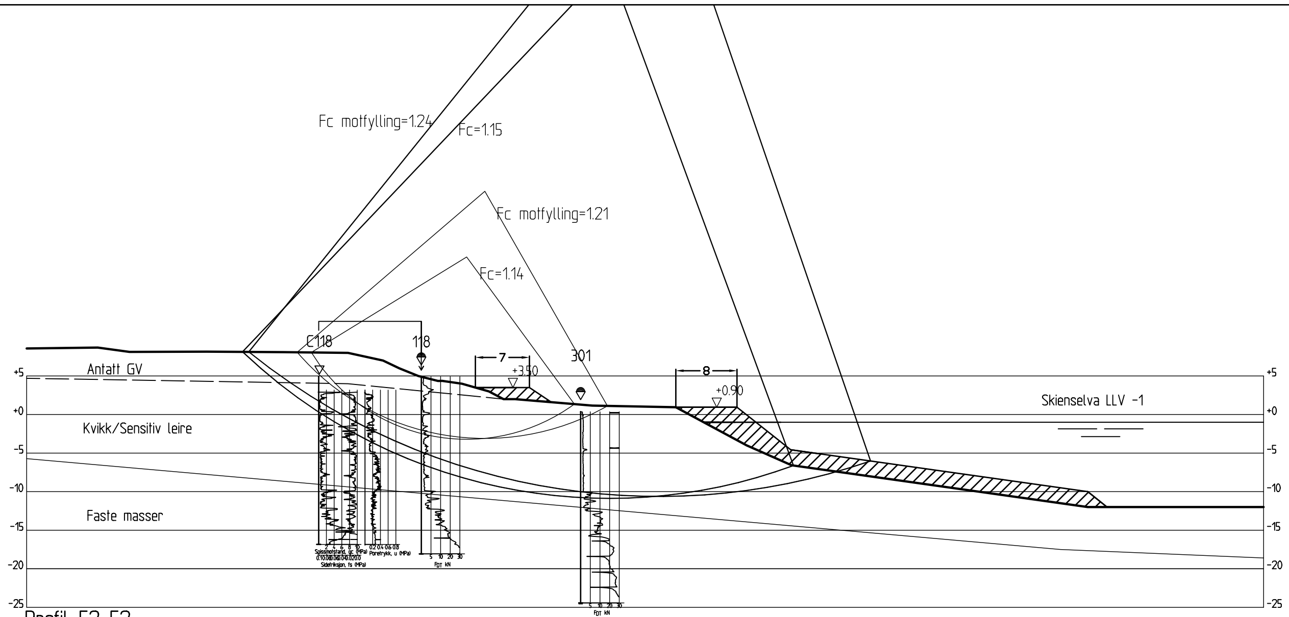
Profil E2-E2 1 : 500
