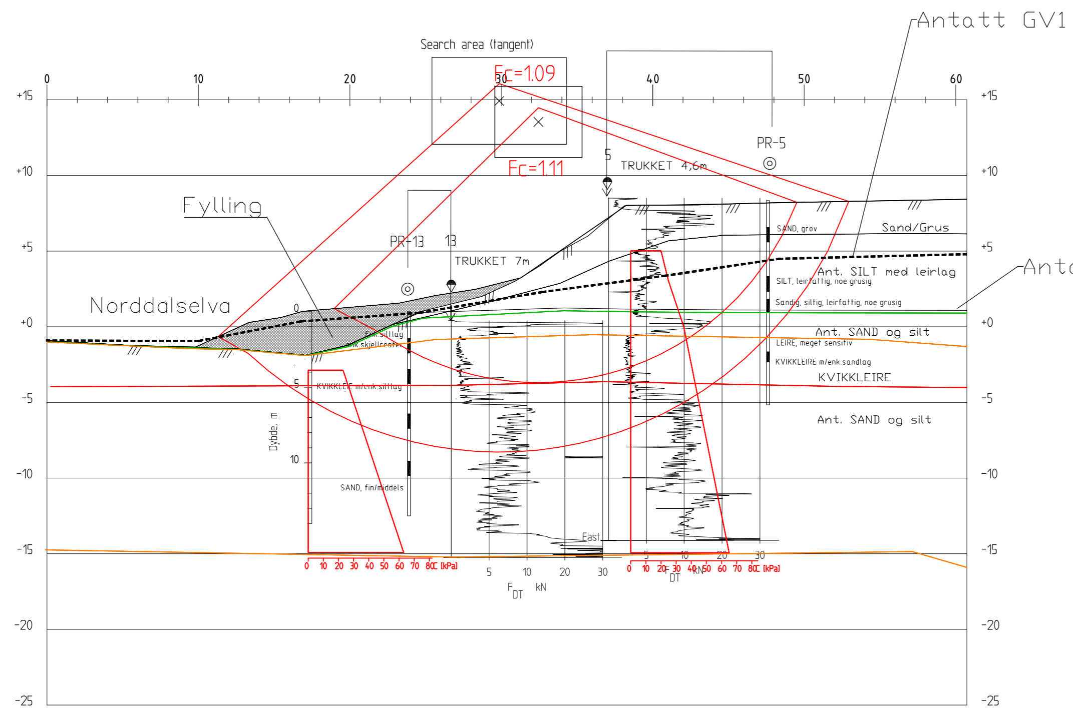
Profil P5-P5 1 : 200
