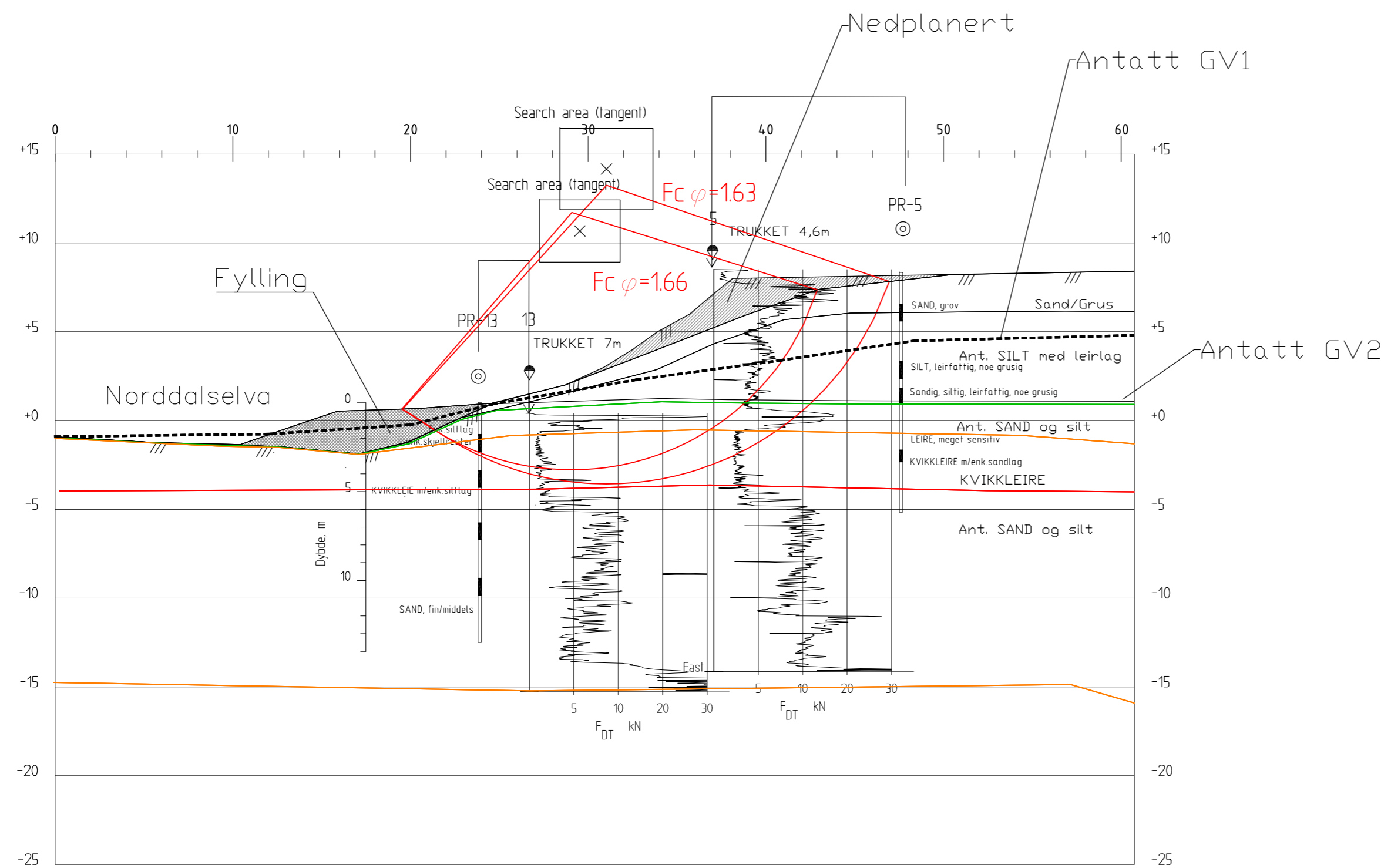
Profil P5-P5 1 : 200
