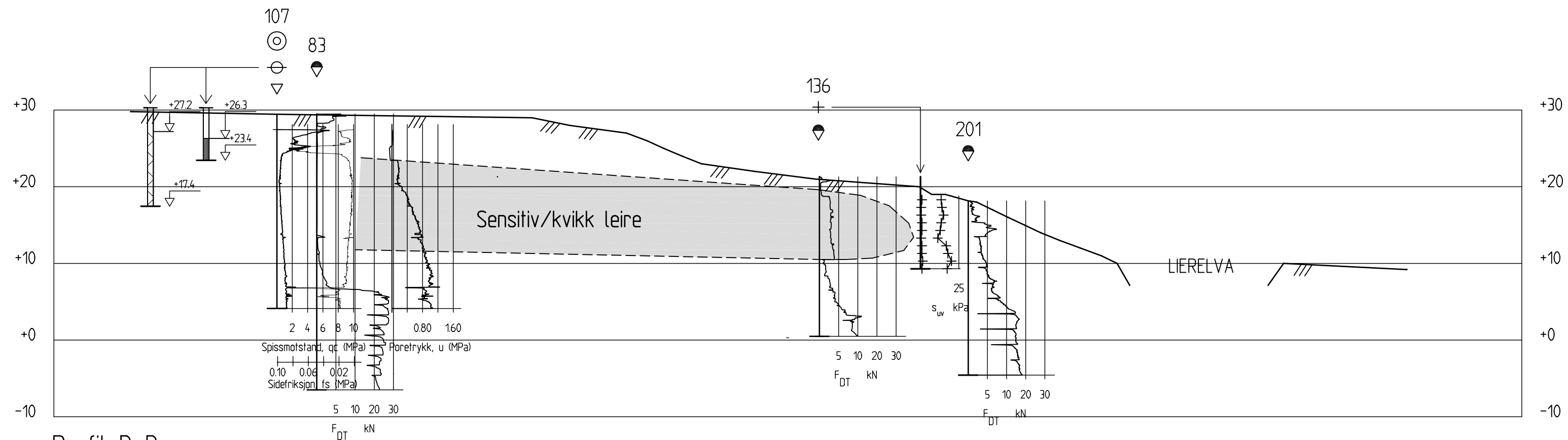
Profil B-B 1 : 500
