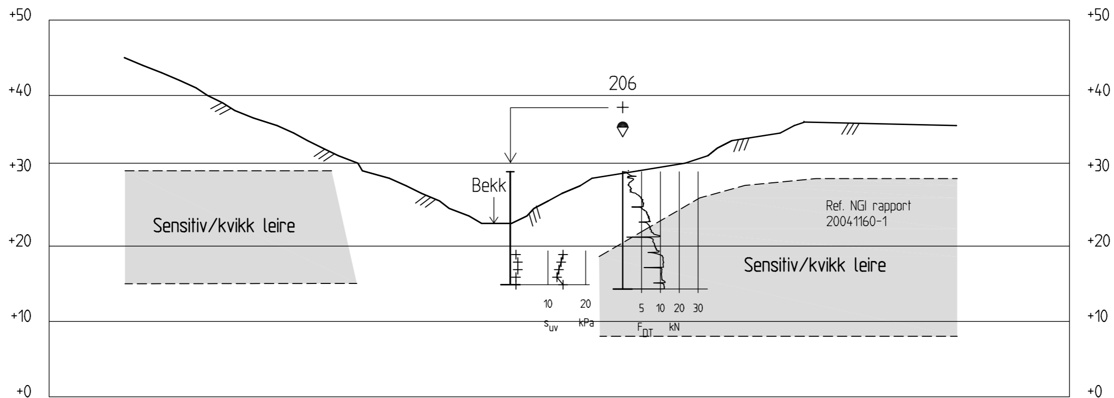
Profil D-D 1 : 500
