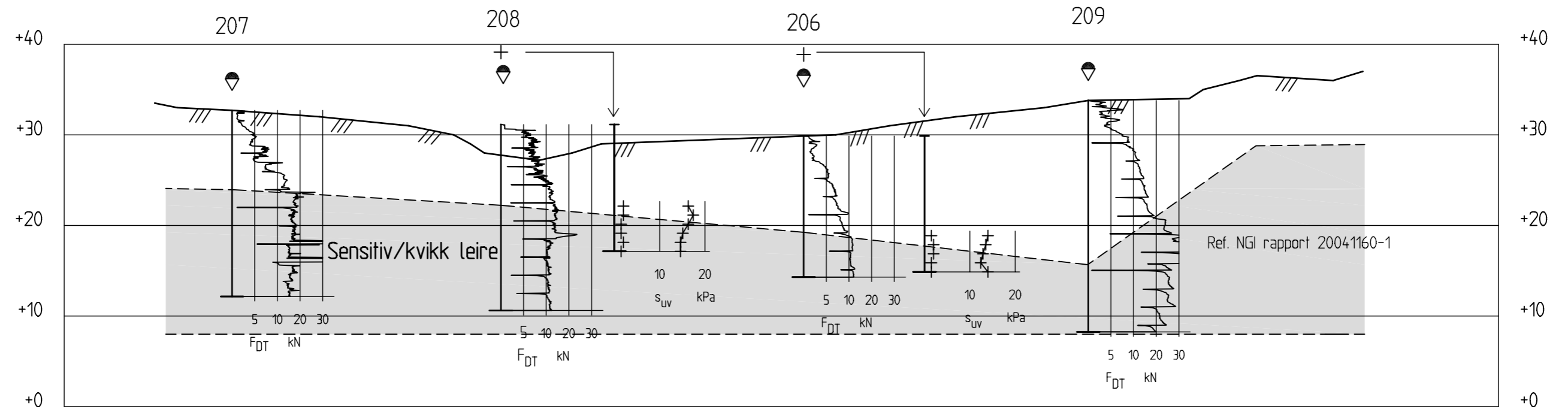
Profil C-C 1 : 500
