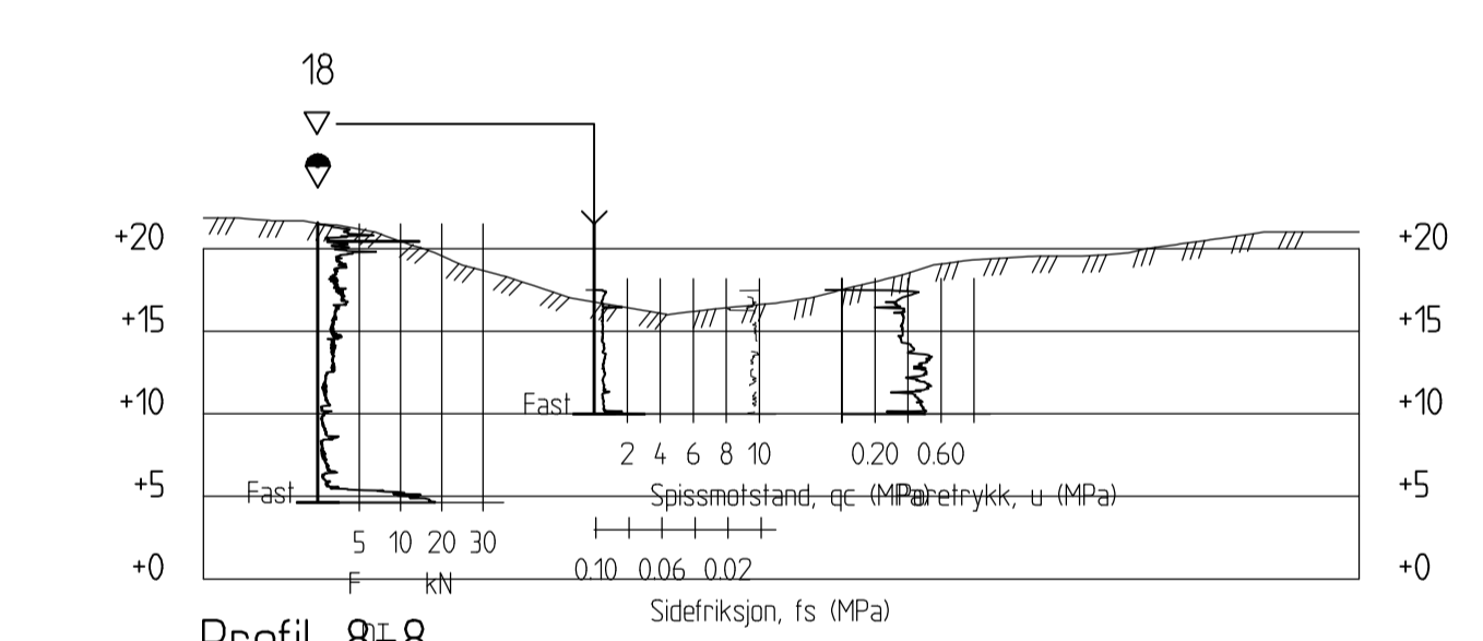
Profil 8+8 1: 500
